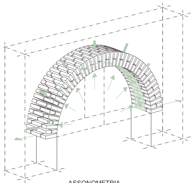
ASSONOMETRIA RINFORZO INTRADOSSALE DELL'ARCO
