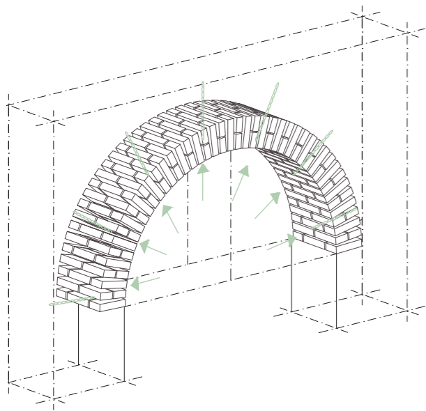
ASSONOMETRIA RINFORZO PUNTUALE DELL'ARCO
