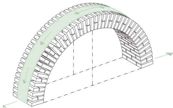
ASSONOMETRIA RINFORZO ESTRADOSSALE DELL'ARCO
