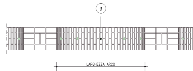
PIANTA B - B' SISTEMI DI RINFORZO ALL'INTRADOSSO CON BARRE ELICOIDALI STEEL DRYFIX® 10
