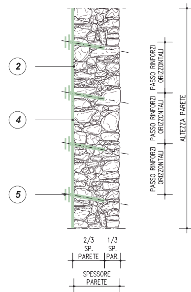
SEZIONE A-A' RINFORZO A FLESSIONE E TAGLIO DEL MASCHIO MURARIO TRAMITE GEOSTEEL G600/G1200 SU UN SOLO LATO DEL PARAMENTO
