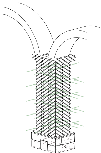
ASSONOMETRIA CONFINAMENTO PUNTUALE DEL PILASTRO CON STEEL DRYFIX® 10
