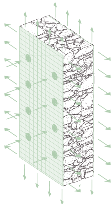
ASSONOMETRIA RETE GEOSTEEL GRID 200/400 O RINFORZO ARV 100
