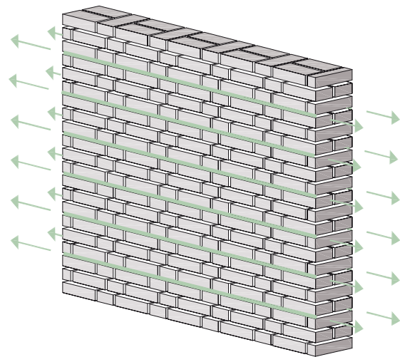
ASSONOMETRIA RISTILATURA ARMATA DEI GIUNTI CON STEEL HELIBAR® 6
