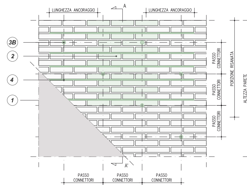
PROSPETTO UNIONE DELL'INTERVENTO DI SCUCI - CUCI CON L'INSERIMENTO DIFFUSO DI CONNESSIONI TRASVERSALI REALIZZATE MEDIANTE BARRE ELICOIDALI STEEL DRYFIX® E RISTILATURA ARMATA CON BARRE ELICOIDALI STEEL HELIBAR® 6
