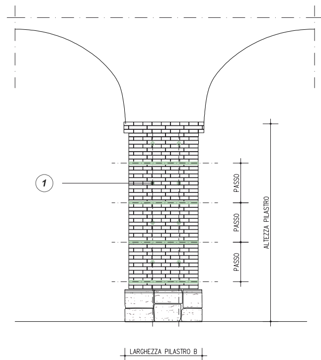
PROSPETTO SEZIONE RETTANGOLARE O QUADRATA CONFINAMENTO PUNTUALE DEL PILASTRO CON STEEL DRYFIX® 10
