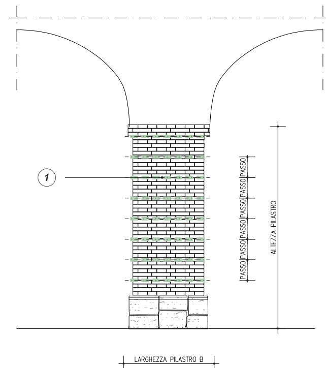
PROSPETTO SEZIONE CIRCOLARE CONFINAMENTO PUNTUALE DEL PILASTRO STEEL DRYFIX® 10
