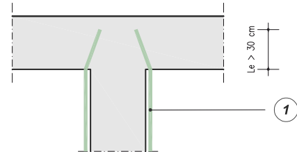
DETTAGLIO 1: ANCORAGGIO SU COLLEGAMENTO A MARTELLO
