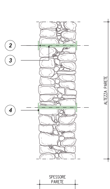
SEZIONE A-A' INSERIMENTO DIFFUSO DI DIATONI ARTIFICIALI A FIOCCO IN FIBRA DI ACCIAIO GALVANIZZATO GEOSTEEL G600/G1200
