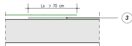
DETTAGLIO 3: LUNGHEZZA DI SOVRAPPOSIZIONE
