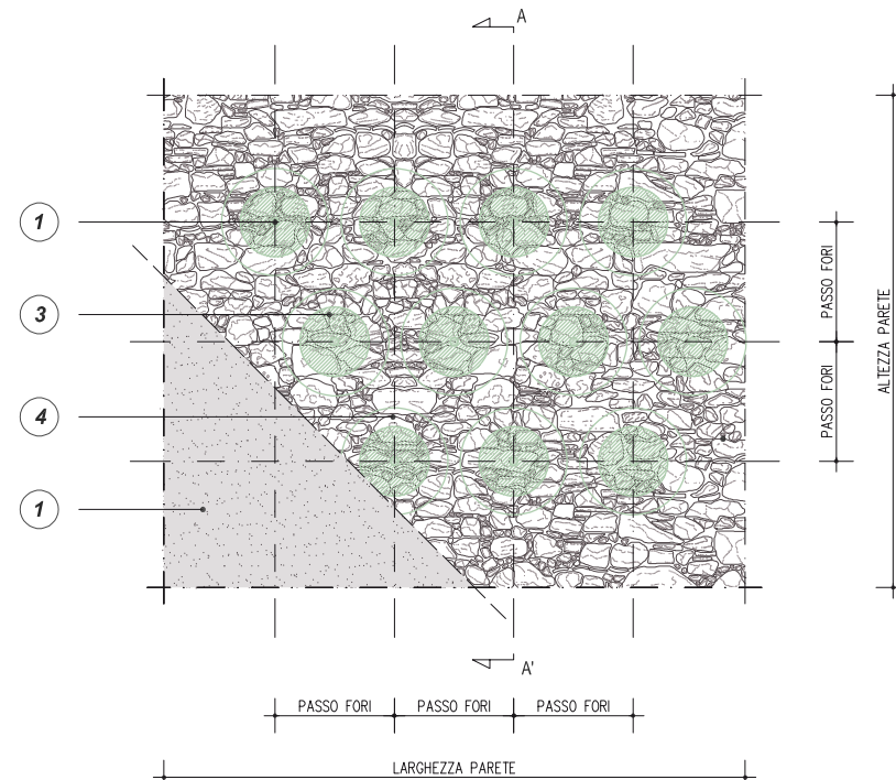
PROSPETTO CONSOLIDAMENTO TRAMITE INIEZIONI DI GEOCALCE® FL ANTISISMICO
