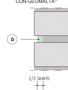
FASE II: PULIZIA E RIEMPIMENTO CON GEOMALTA®
