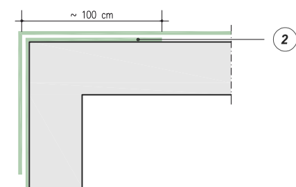
DETTAGLIO 2: ANCORAGGIO SUI CANTONALI
