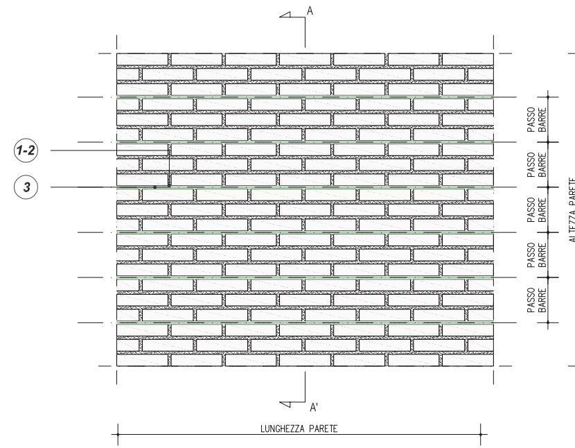
PROSPETTO INTERVENTO DI RISTILATURA ARMATA DEI GIUNTI CON STEEL HELIBAR® 6
