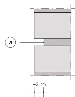
FASE I: SCARNIFICAZIONE DEL GIUNTO
