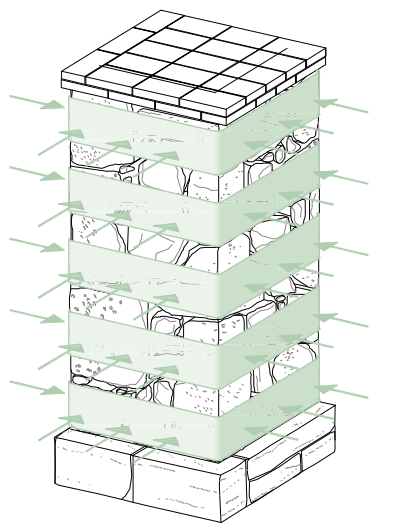
ASSONOMETRIA CONFINAMENTO DEL PILASTRO CON GEOSTEEL G600/G1200
