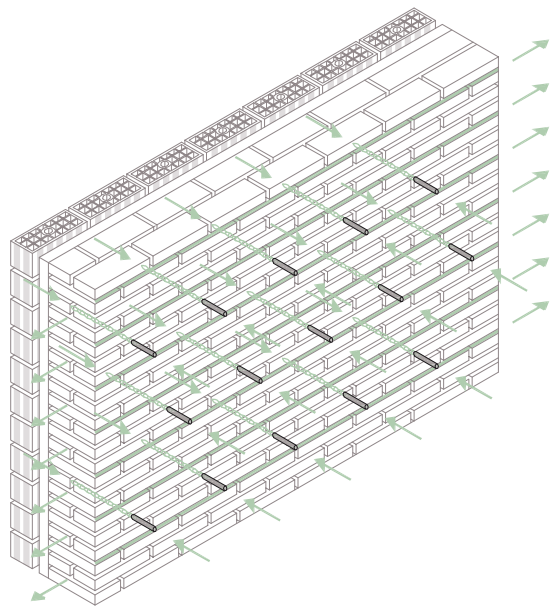
ASSONOMETRIA RISTILATURA ARMATA DEI GIUNTI CON STEEL HELIBAR® 6
