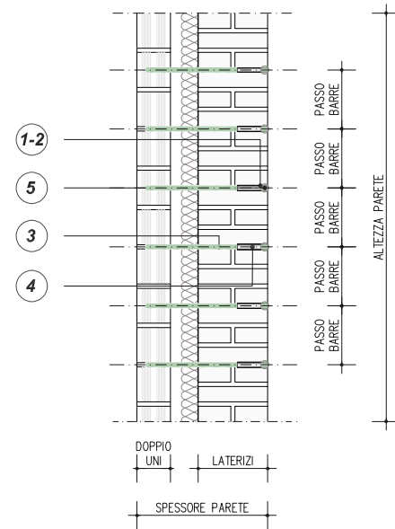
SEZIONE A-A' INTERVENTO DI RISTILATURA ARMATA DEI GIUNTI TRAMITE STEEL HELIBAR® 6 E CONNESSIONI TRASVERSALI CON STEEL DRYFIX® 10 E CONNETTORE STEEL DRYFIX® 10
