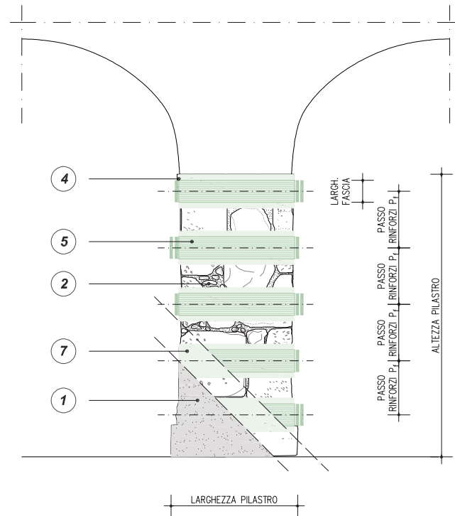
PROSPETTO CONFINAMENTO DEL PILASTRO MEDIANTE FASCIATURA DISCONTINUA CON GEOSTEEL G600/G1200
