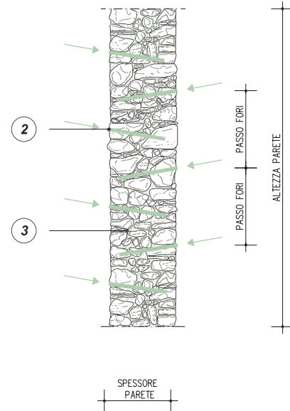
SEZIONE A-A' CONSOLIDAMENTO TRAMITE INIEZIONI DI GEOCALCE® FL ANTISISMICO
