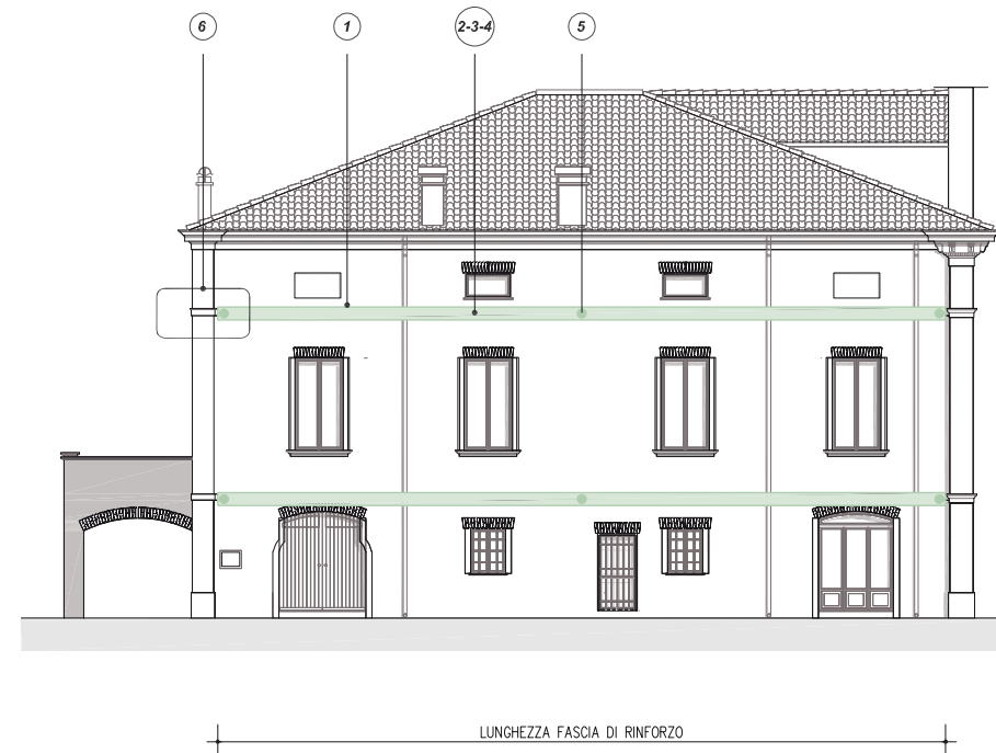
PROSPETTO B-B' RINFORZO DI PORZIONI DI FABBRICATO MEDIANTE FASCE GEOSTEEL G600/G1200
