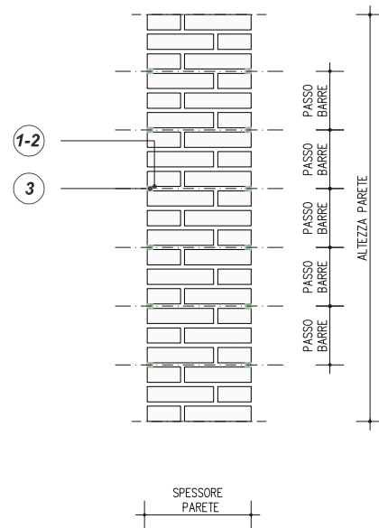
SEZIONE A-A' INTERVENTO DI RISTILATURA ARMATA DEI GIUNTI CON STEEL HELIBAR® 6
