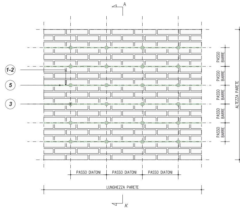
PROSPETTO INTERVENTO DI RISTILATURA ARMATA DEI GIUNTI TRAMITE STEEL HELIBAR® 6 E CONNESSIONI TRASVERSALI CON STEEL DRYFIX® 10 E CONNETTORE STEEL DRYFIX® 10
