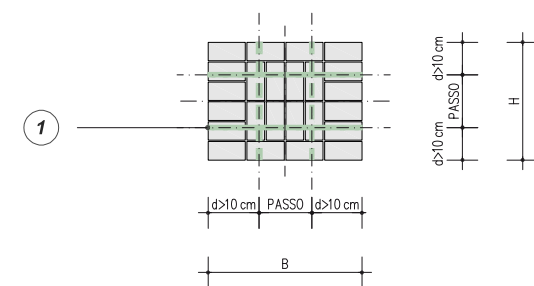
PIANTA SEZIONE RETTANGOLARE CONFINAMENTO PUNTUALE DEL PILASTRO CON STEEL DRYFIX® 10
