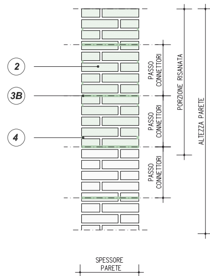
SEZIONE A-A' UNIONE DELL'INTERVENTO DI SCUCI - CUCI CON L'INSERIMENTO DIFFUSO DI CONNESSIONI TRASVERSALI REALIZZATE MEDIANTE BARRE ELICOIDALI STEEL DRYFIX® E RISTILATURA ARMATA CON BARRE ELICOIDALI STEEL HELIBAR® 6
