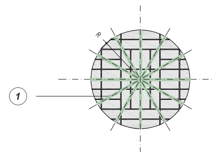
PIANTA SEZIONE CIRCOLARE CONFINAMENTO PUNTUALE DEL PILASTRO CON STEEL DRYFIX® 10
