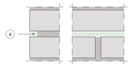
FASE III: INSERIMENTO STEEL HELIBAR® 6
