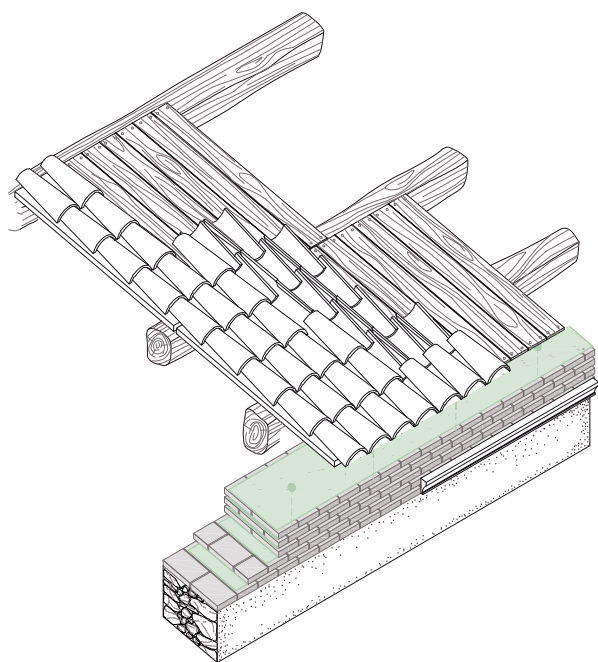
ASSONOMETRIA CORDOLO IN MURATURA ARMATA
