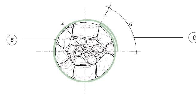
PIANTA SEZIONE CIRCOLARE CONFINAMENTO DEL PILASTRO MEDIANTE FASCIATURA DISCONTINUA CON GEOSTEEL G600/G1200
