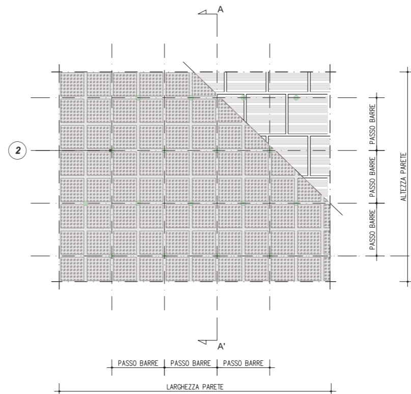
PROSPETTO CUCITURA A SECCO CON STEEL DRYFIX® 10 DI INTONACI IN GROSSO SPESSORE O DI RIVESTIMENTI DI FACCIATA
