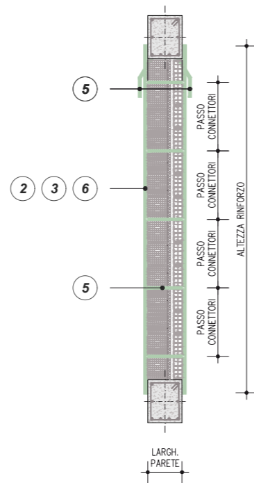
SEZIONE A-A' SISTEMA DI PRESIDIO ANTIRIBALTAMENTO DELLA TAMPONATURA TRAMITE GEO GRID 120 E BARRE STEEL DRYFIX 10 EFFETTUATO SU ENTRAMBI I LATI DEL PARAMENTO
