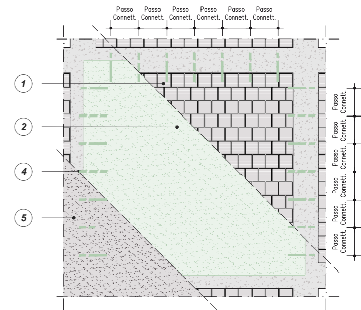
INTERVENTO AGGIUNTIVO 2 PRESIDIO ANTIRIBALTAMENTO MEDIANTE INTONACO TECNICO COMPOSITO GEOCALCE® TENACE E INSTALLAZIONE A SECCO BARRE STEEL DRYFIX 10
