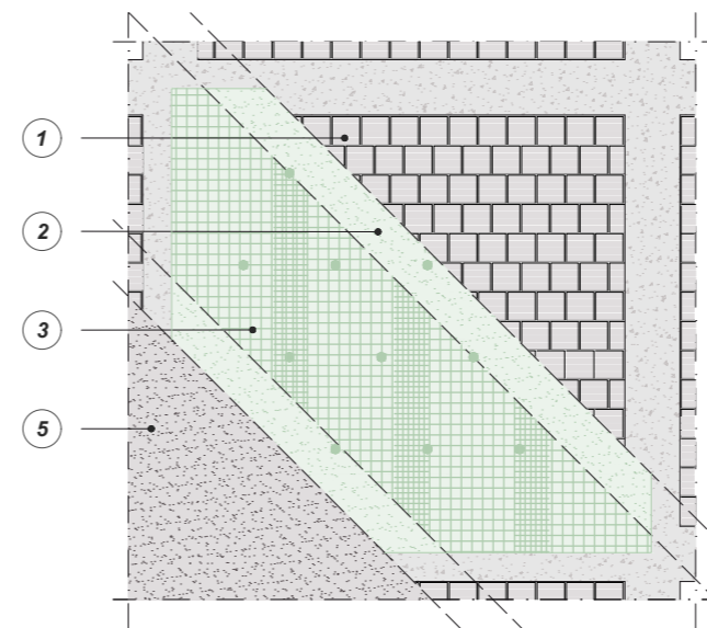
INTERVENTO AGGIUNTIVO 1 PRESIDIO ANTIRIBALTAMENTO MEDIANTE INTONACO TECNICO COMPOSITO GEOCALCE® TENACE E GEO GRID 120
