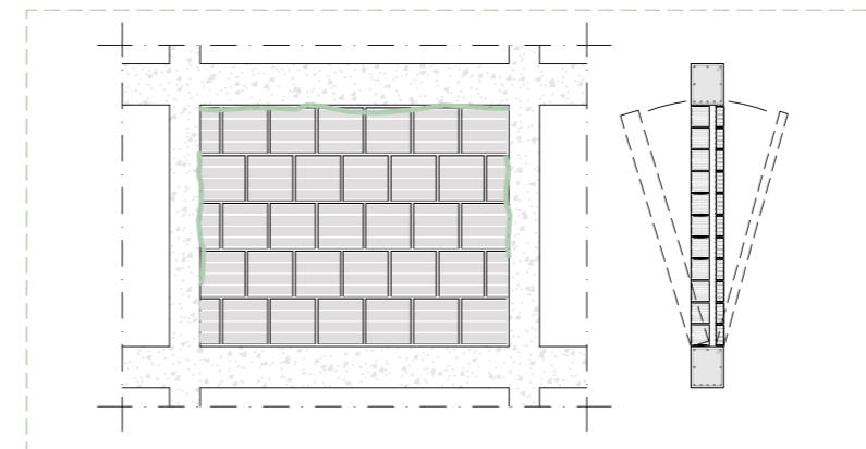
MECCANISMO DI COLLASSO 2
