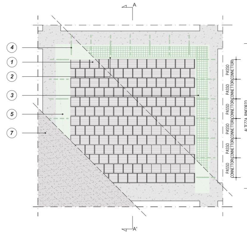
PROSPETTO RINFORZO DELLA TAMPONATURA TRAMITE GEO GRID 120 IN ABBINAMENTO A GEOCALCE F ANTISISMICO E BARRE ELICOIDALI IN ACCIAIO INOX
