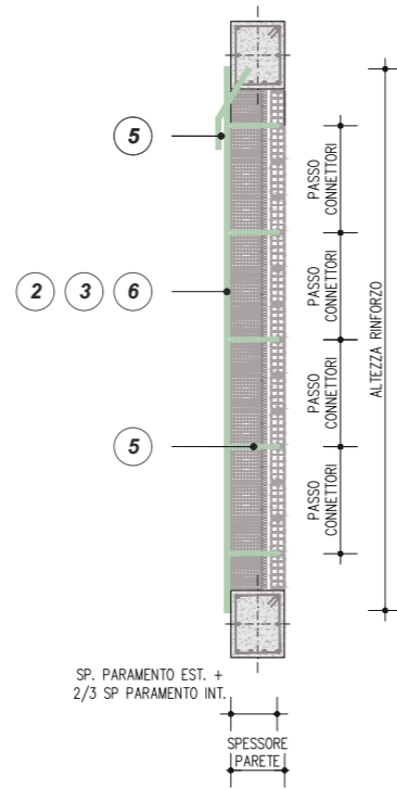
SEZIONE A-A' SISTEMA DI PRESIDIO ANTIRIBALTAMENTO DELLA TAMPONATURA TRAMITE GEO GRID 120 E BARRE STEEL DRYFIX 10 EFFETTUATO SU UN SOLO LATO DEL PARAMENTO
