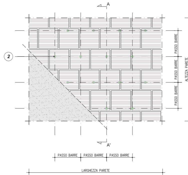
PROSPETTO CUCITURA A SECCO CON STEEL DRYFIX® 10 DI TAMPONATURE A DOPPIO PARAMENTO
