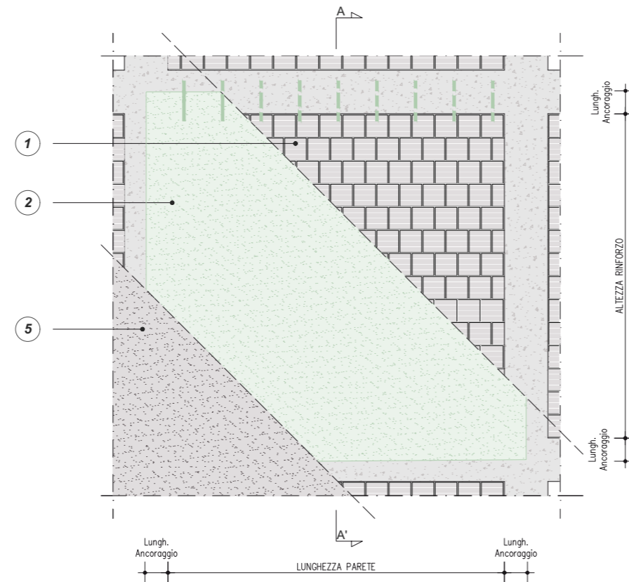
PIANTA PRESIDIO ANTIRIBALTAMENTO MEDIANTE INTONACO TECNICO COMPOSITO GEOCALCE® TENACE
