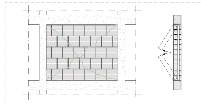
MECCANISMO DI COLLASSO 1
