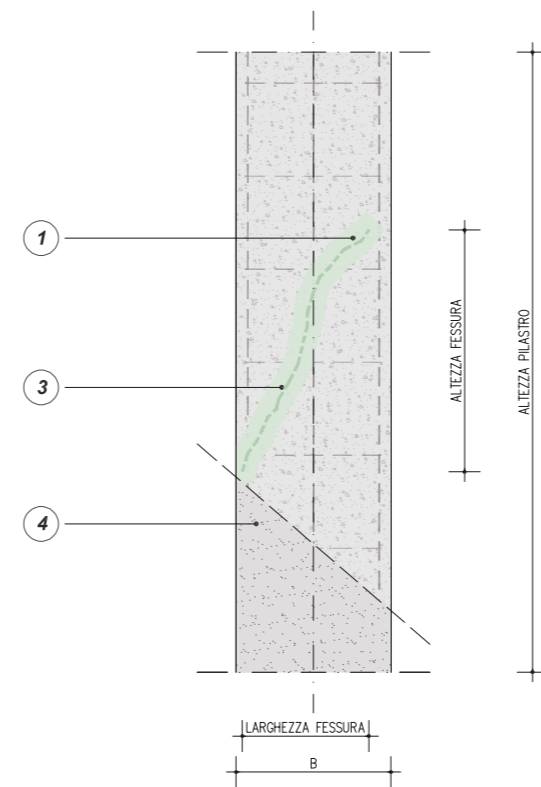
PROSPETTO RIPARAZIONE/RICUCITURA DI FESSURE MEDIANTE STUCCATURA CON RESINA
