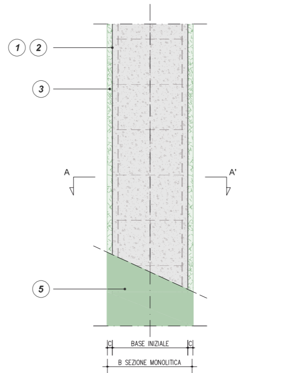
PROSPETTO DEL PILASTRO RINFORZO MEDIANTE RICOSTRUZIONE VOLUMETRICA MONOLITICA DELLA SEZIONE CON SISTEMI GEOLITE® FRC
