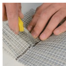
Sfocchettatura tessuto Geosteel
