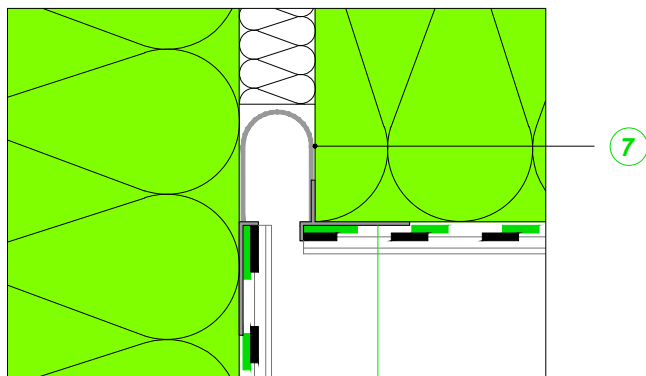
DETALLE A
